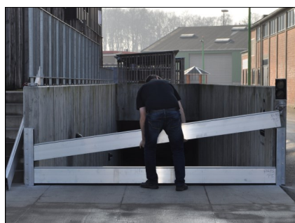
Bjælkerne, der beskytter P-kælderen, lægges hurtigt til rette mellem de fastmonterede profiler. De er ca. 325 cm lange og vejer hver kun 13,4 kg.
